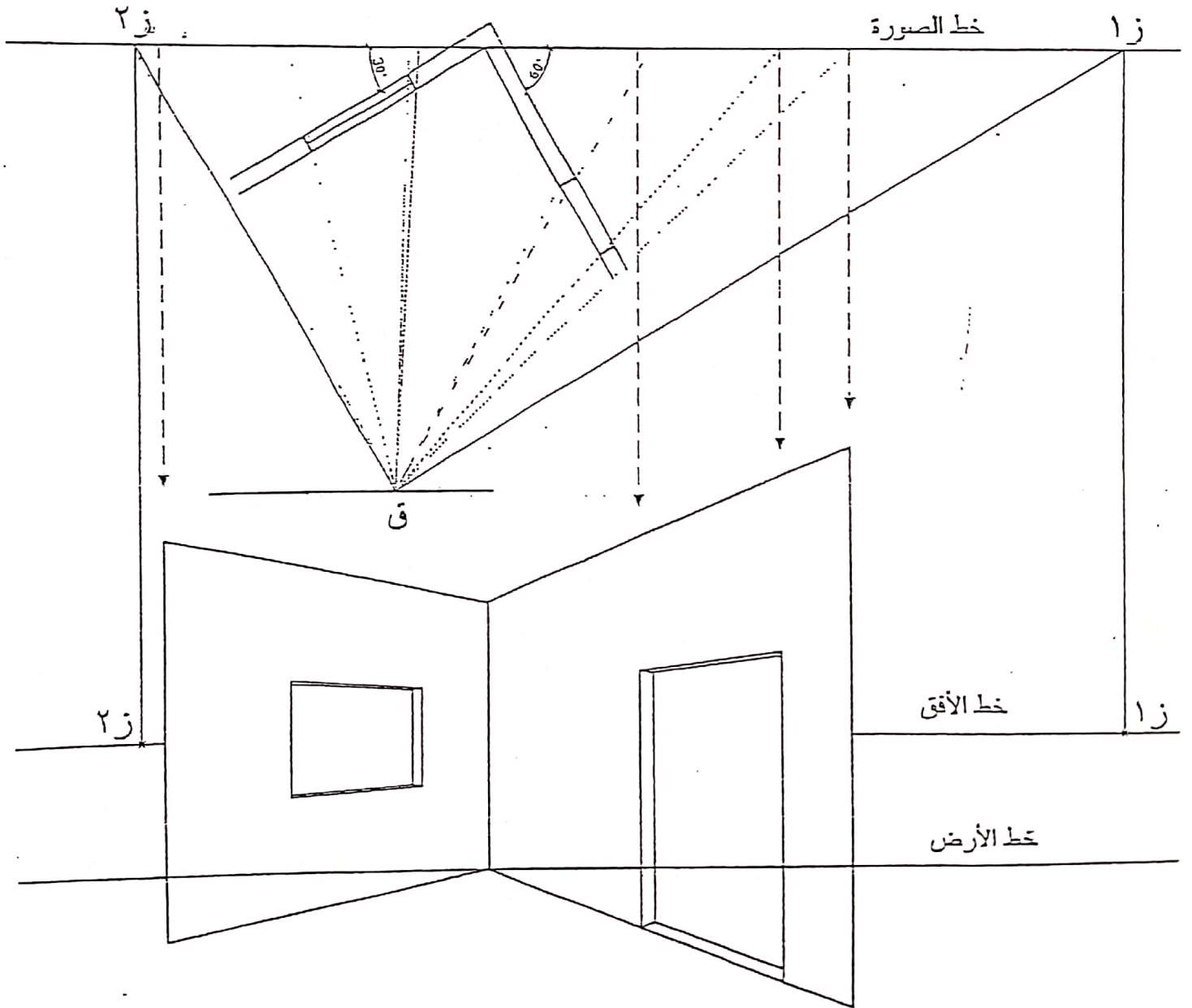
شكل (٣٣) منظور بنقطتي تلاشي لغرفة أمام خط الصورة
